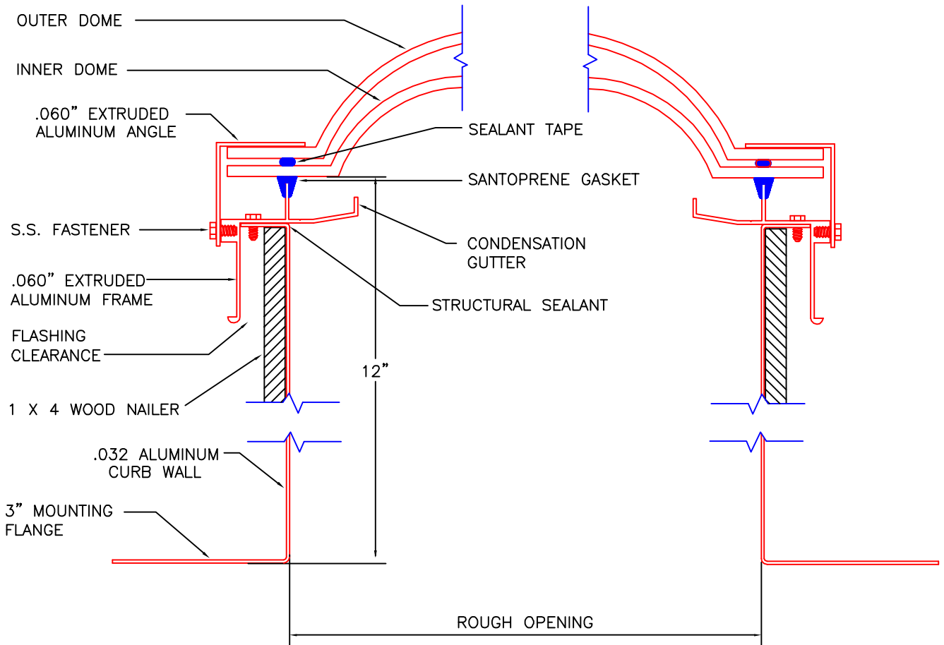
12" EZ SELF FLASHING (MODEL EZSF-12)
